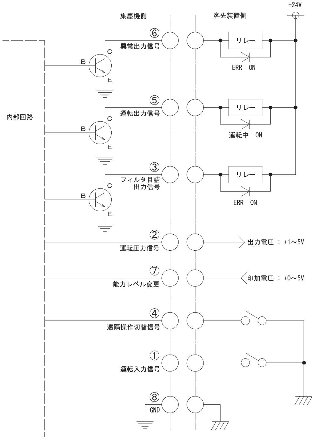
図6.1 リモートの標準接続図
