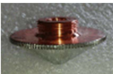
Φ28の噴射ノズル
